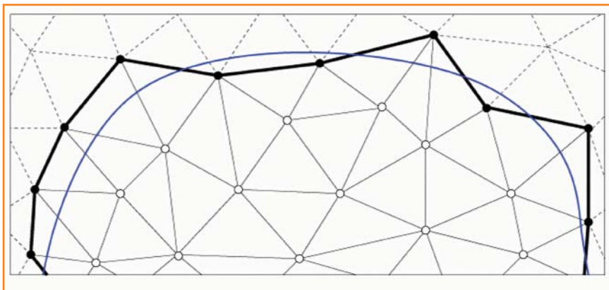
Figura 7 – As arestas apontadas representam as arestas interiores da malha-d conectando dois vértices marcados. A fronteira da malha-d está desenhada com segmentos grossos e a linha curva representa a fronteira do modelo. Para facilitar a visualização, a malha-d está representada em duas dimensões, mas o caso para três dimensões é análogo.
