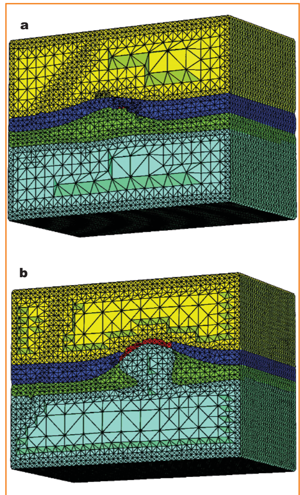
Figura 19a,b – Corte da malha do domo de sal.
