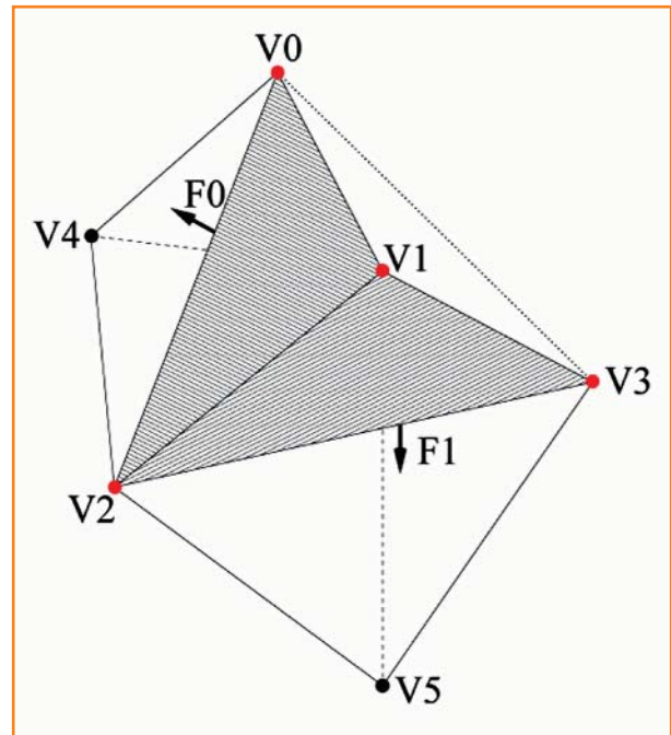
Figura 11 – Tetraedro exterior com os quatro vértices marcados: V_0 , V_1 , V_2 , e V_3 . As faces de fronteira são as hachuradas ( F_0 e F_1 ) e as setas apontam para o interior do modelo.
